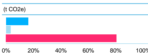
Fig. 2 : Répartition des émissions en pourcentage.
