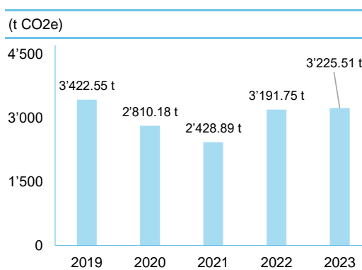
Fig. 1 : Émissions totales des cinq dernières années, de 2019 - 2023
